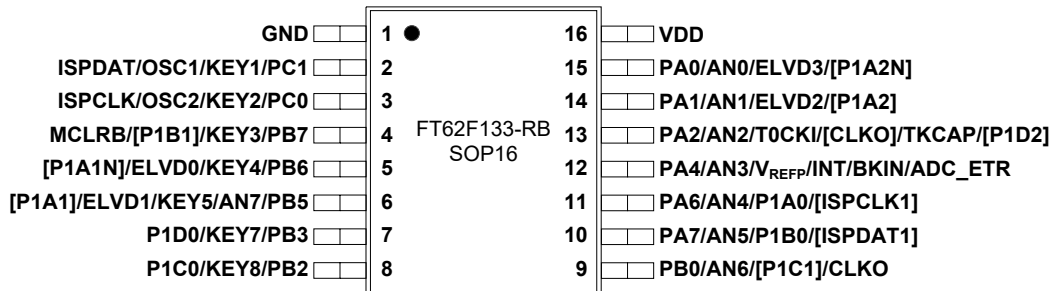
图 1-5 SOP16 1
