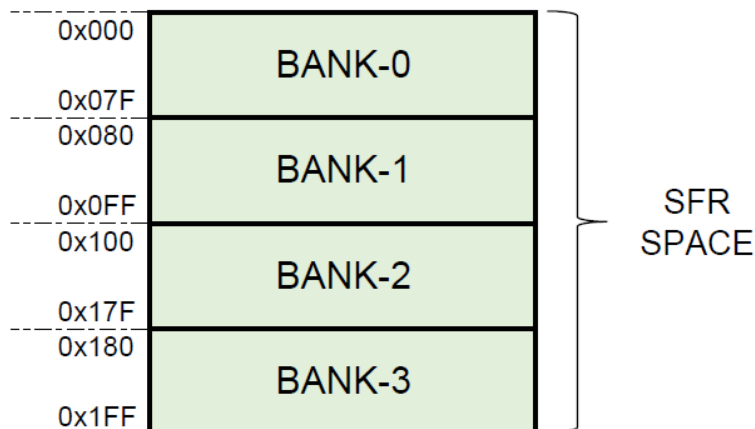
图 17-2 间接寻址
