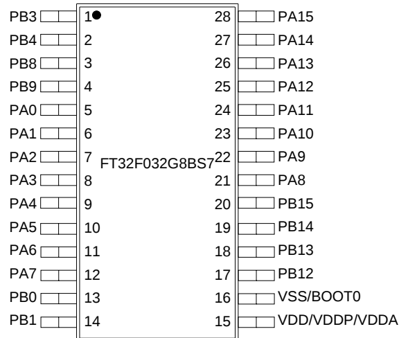
图 4-5 SOP28 引脚分配
