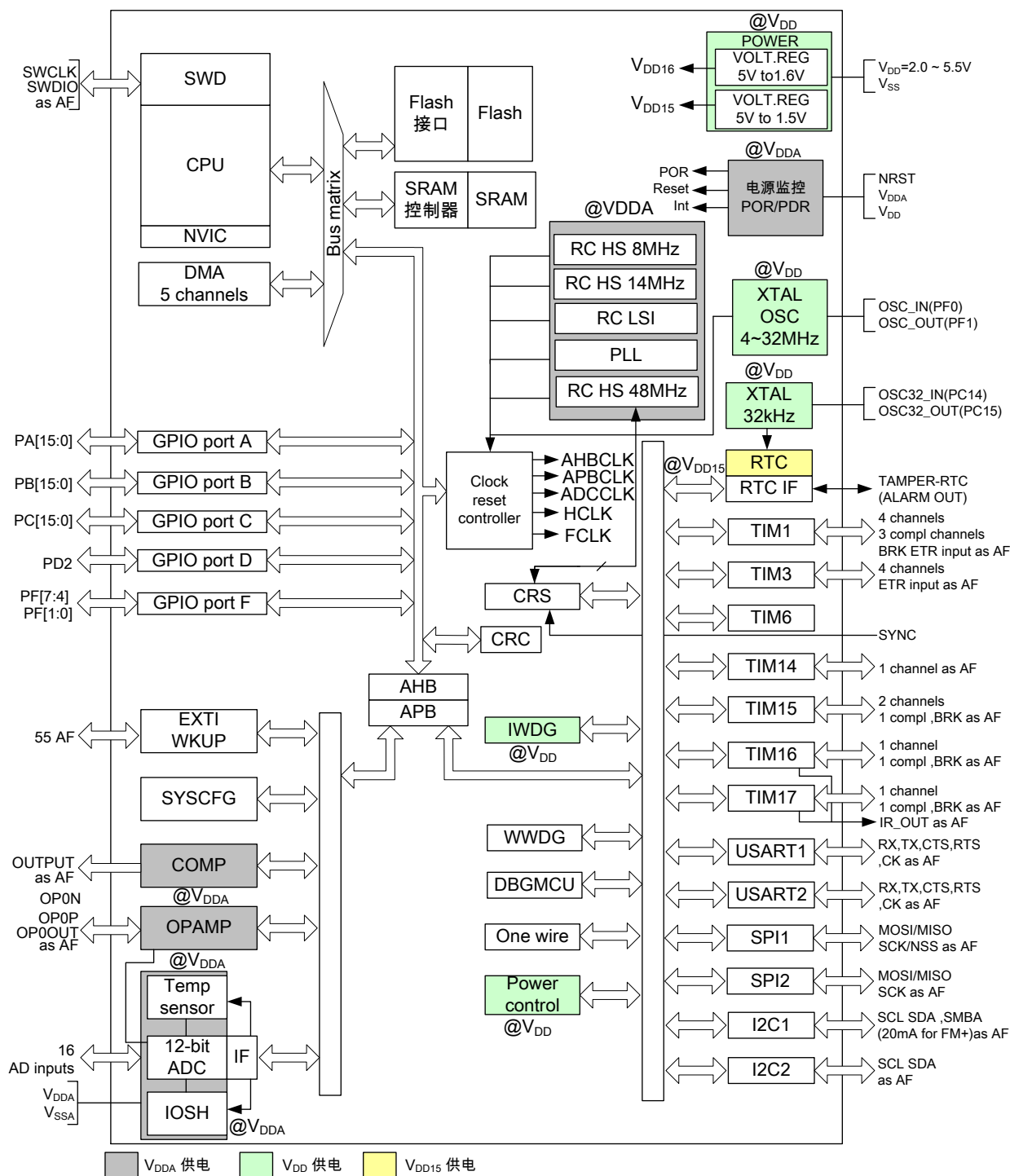
图 2-1 系统框图
