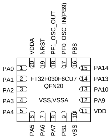
图 4-10 QFN20 引脚分配 6
