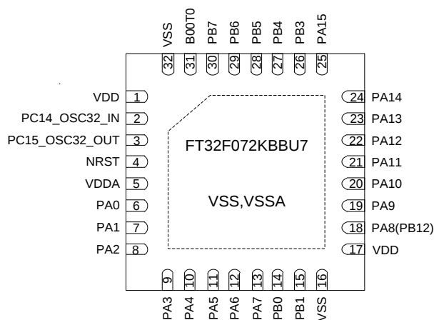
图 4.4 QFN32-B 引脚分配
