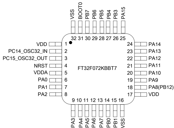
图 4.3 LQF32 引脚分配
