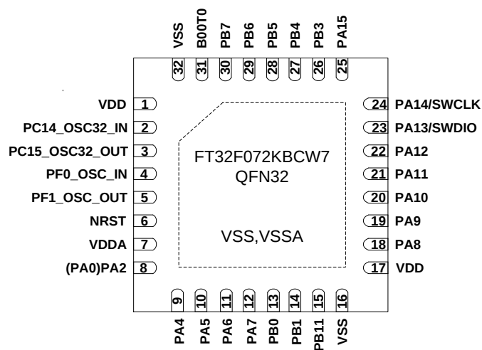
图 4.5 QFN32-C 引脚分配
