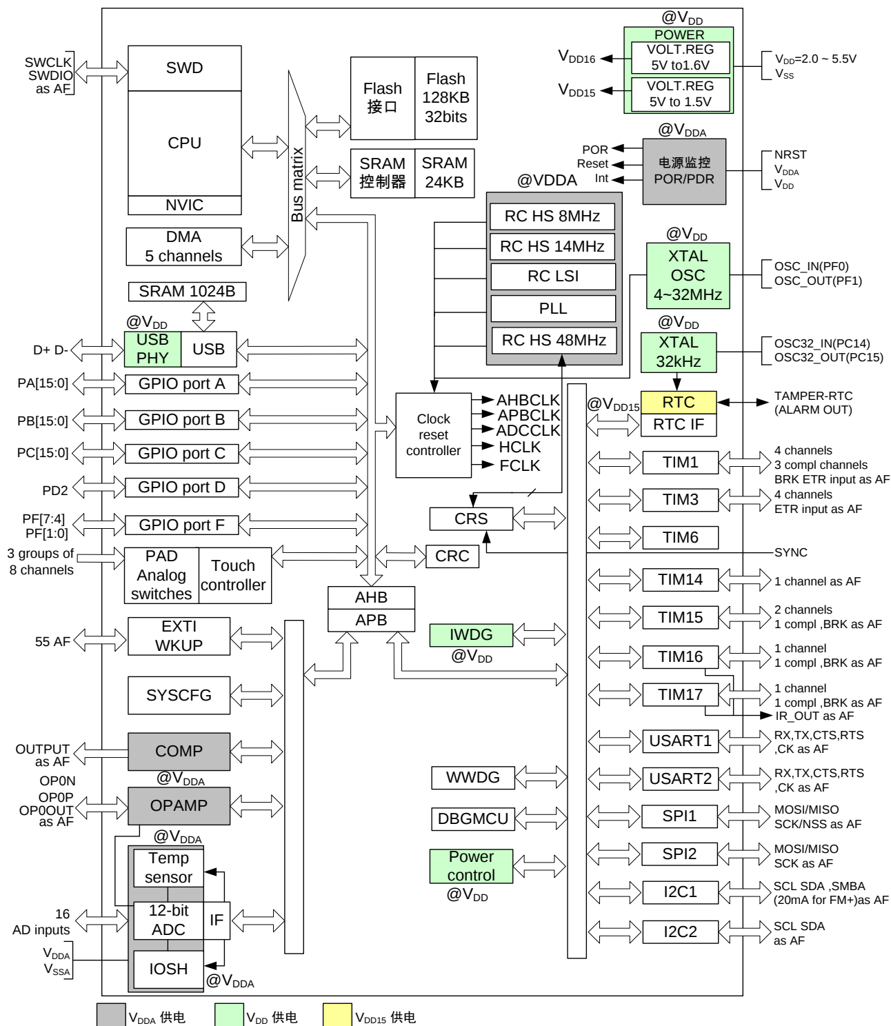
图 2.1 系统框图
