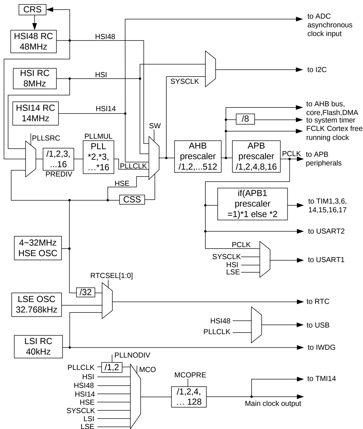
图 3.1 时钟框图
